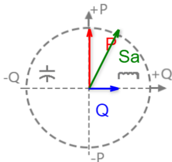
Рисунок 17 – Диаграмма полной мощности
