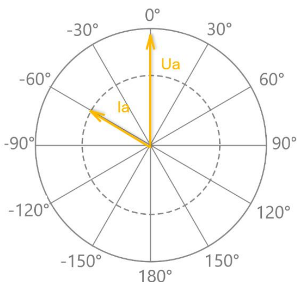
Рисунок 16 – Векторная диаграмма токов и напряжений
