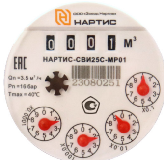
Рисунок 2 – Индикаторное устройство счетчика НАРТИС-СВИ
