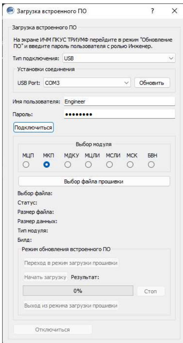
Рис. 1 Главное окно приложения
