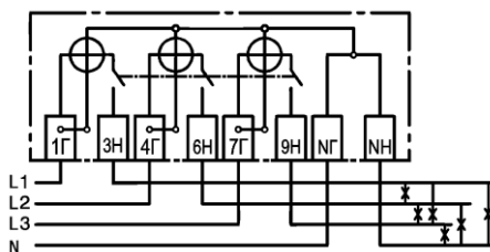
Рисунок 5 – Маркировка схемы включения счетчика «НАРТИС-ИЗ00» архитектуры «Сплит»
