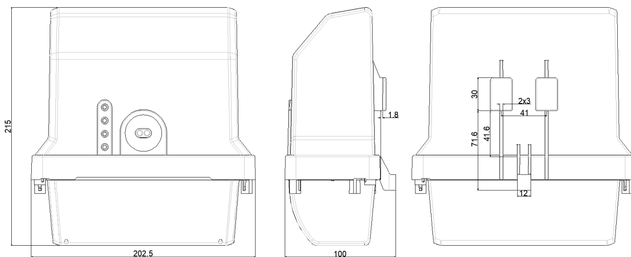
Рисунок 10 – Габаритные и присоединительные размеры счетчика архитектуры «Сплит»
