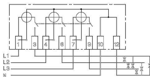
Рисунок 4 – Маркировка схемы включения счетчика «НАРТИС-ИЗ00»
