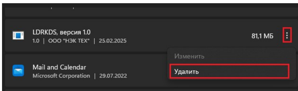
Рис. 15 Удаление приложения
