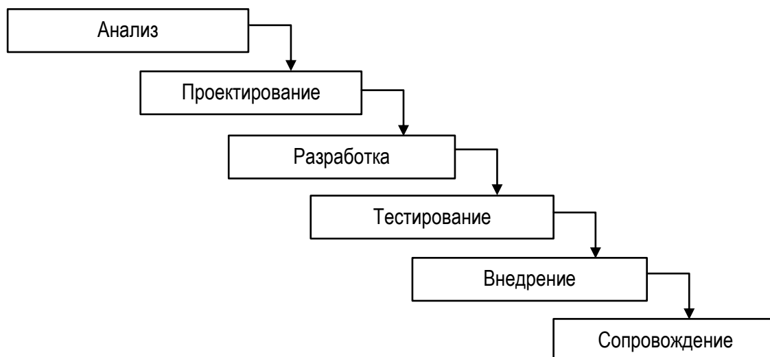
Рисунок 5.1 – Модель ЖЦ
